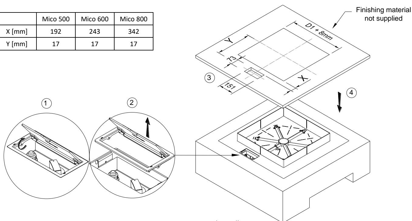
Fig. 4 – Optional installation
